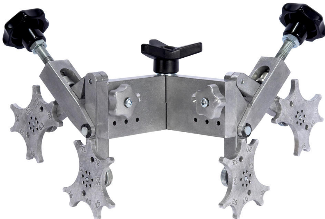
Позиционер д.16-63
