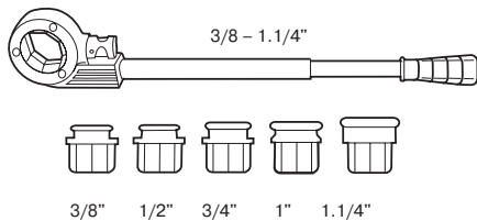
Рукоятка № 6000021
