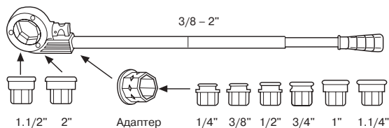
Рукоятка № 6010121
